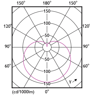
LEDbulb 17.5-150W A67 E27
