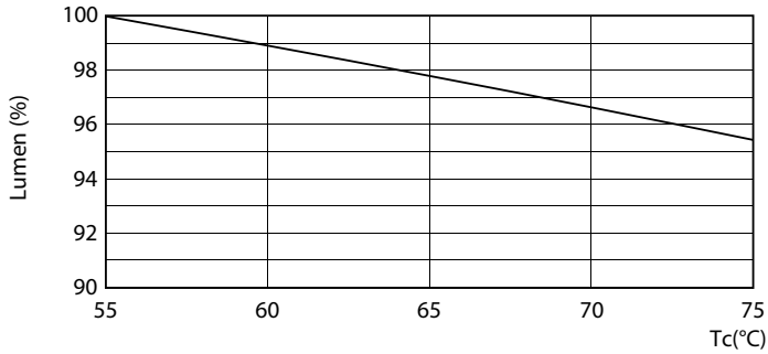
TLED_220-240V_G13-LumenVsTc
