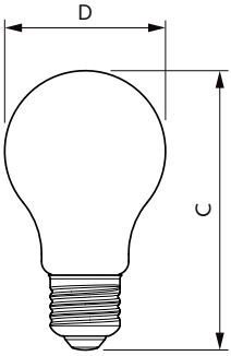
MASTER VLE LEDBulb DT7.2-75W E27 927A60CL G
