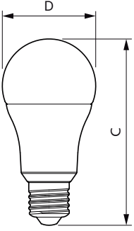
Bulb A65 HV 13-W 1350lm 3000K E27 ND FR
