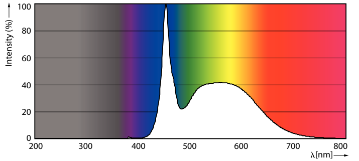
26W G5
