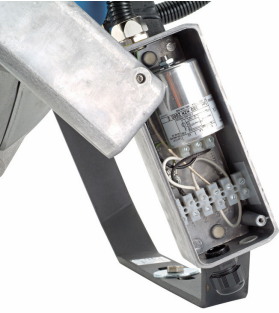
Seri ateşleyiciler içeren elektrik bağlantı kutusu
